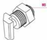
Vite con innesto in cava M8 e dado Cod.W023C (33)
