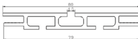
Profilo in alluminio per fissaggio tela a M081 Cod.M0811
