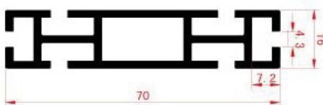
Profilo 6 cave/70 mm
