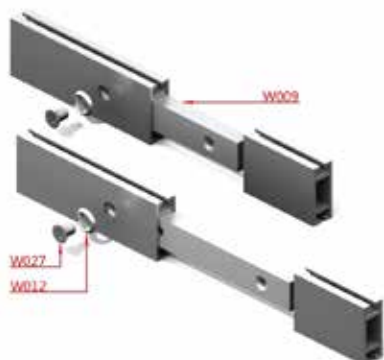
Giunto trasversino Cod.W009
