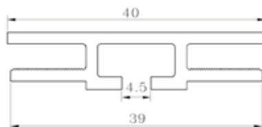
Profilo in alluminio per fissaggio tela a M041 Cod.M043
