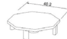
Tappo plastica per S011 - S012 - S013 Cod.SP001
