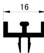
Profilo inferiore ante scorrevoli Cod.E002
