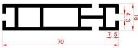
Profilo quattro cave/70 mm
