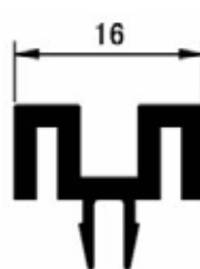
Profilo inferiore ante scorrevoli Cod.E020
