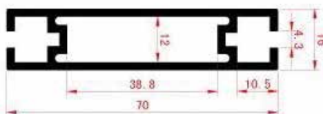
Profilo due cave/70 mm
