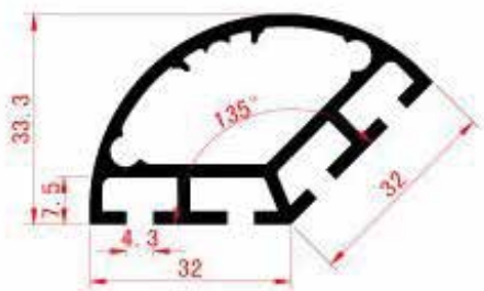
Profilo angolare 135° 4 vie
