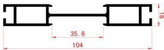
Profilo doppia trave 140 mm
