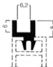
Profilo in plastica per fissaggio Cod.E010
