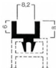
Profilo in plastica per fissaggio Cod.E009
